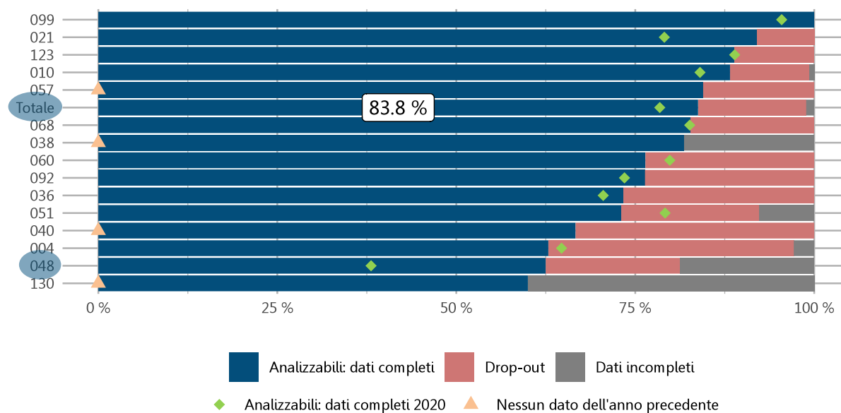
Figura 4: esempi di lettura per i tipi di grafico utilizzati: diagramma a barre – qualità dei dati
