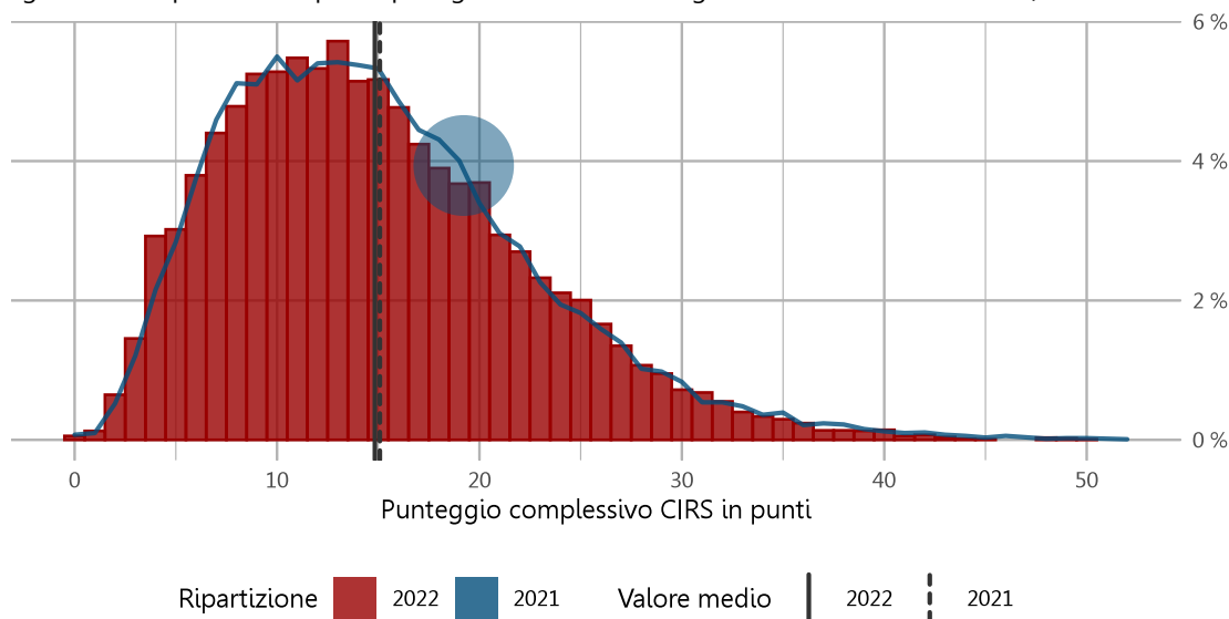
Figura 5: esempi di lettura per i tipi di grafico utilizzati: istogramma – variabili metriche (confronto annuale)
