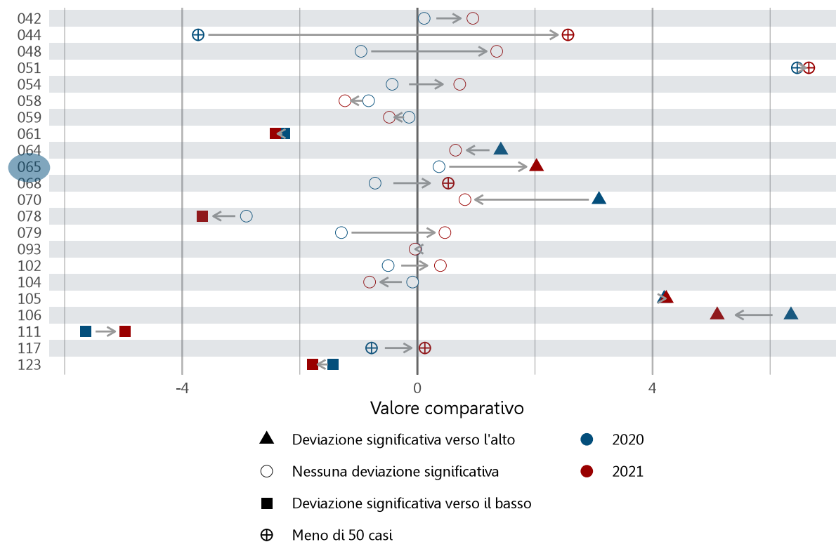
Figura 10: esempi di lettura per i tipi di grafico utilizzati: diagramma di dumbbell – valori comparativi nel confronto annuale
