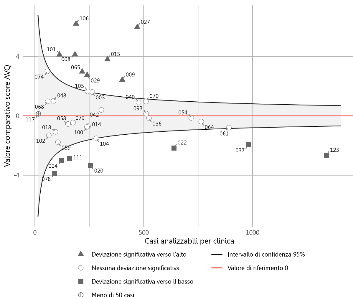
Figura 2: grafico a imbuto – grafico modello
