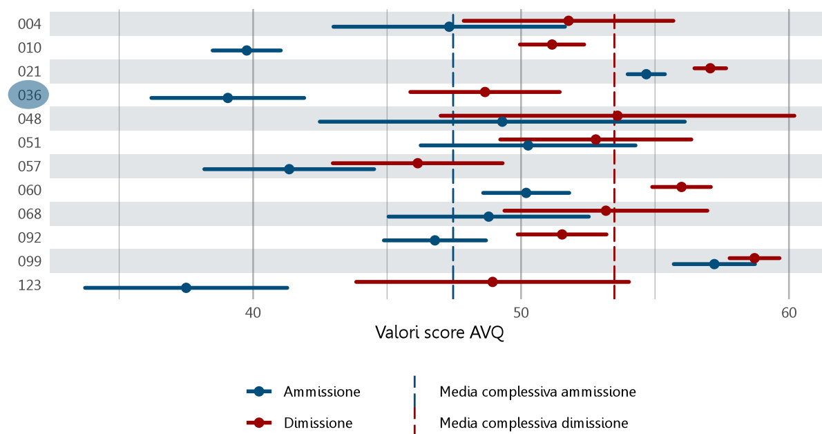
Figura 8: esempi di lettura per i tipi di grafico utilizzati: diagramma a barre di errore – altri indicatori dei risultati (non aggiustati)
