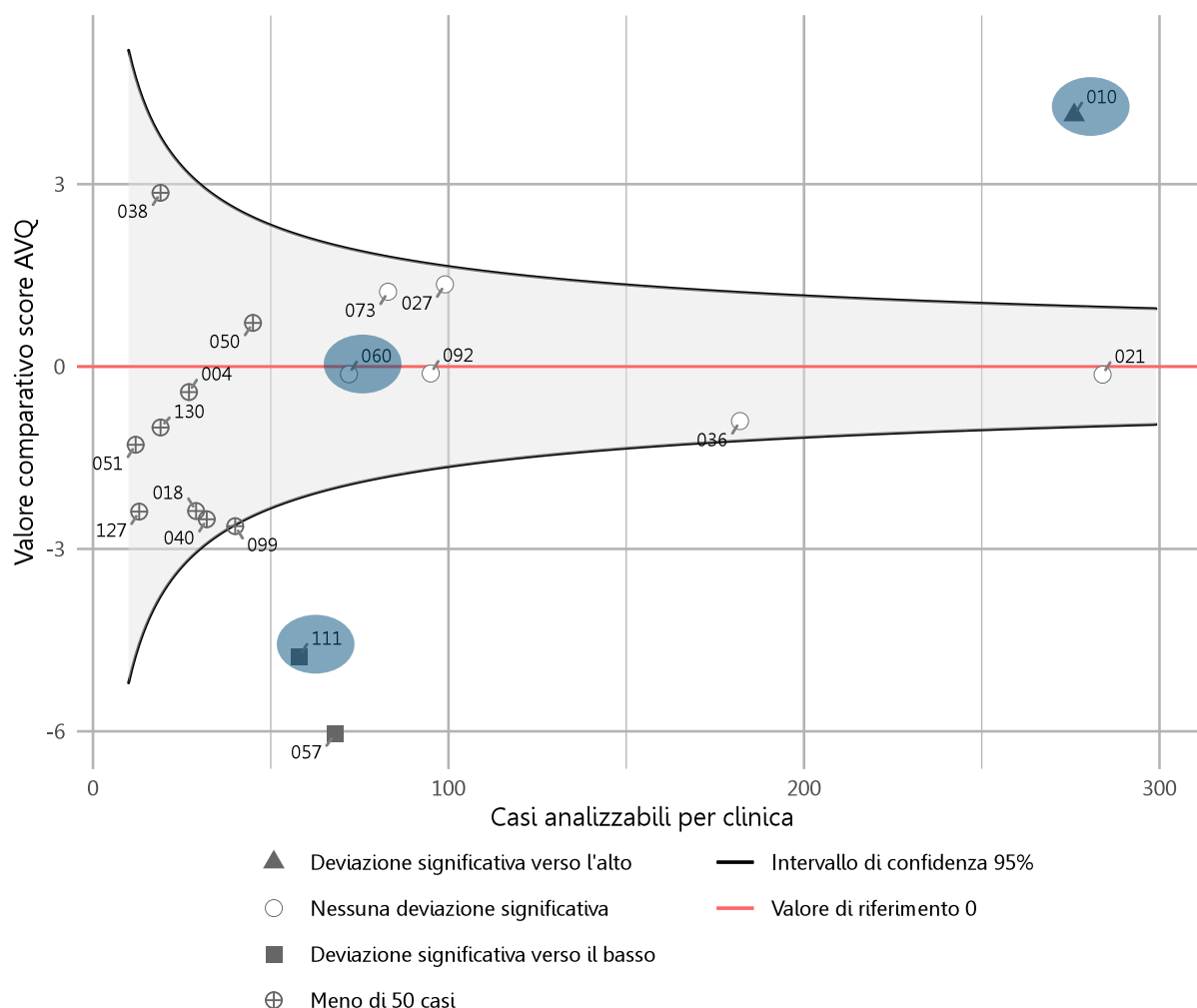
Figura 9: esempi di lettura per i tipi di grafico utilizzati: grafico a imbuto – valori comparativi degli indicatori dei risultati
