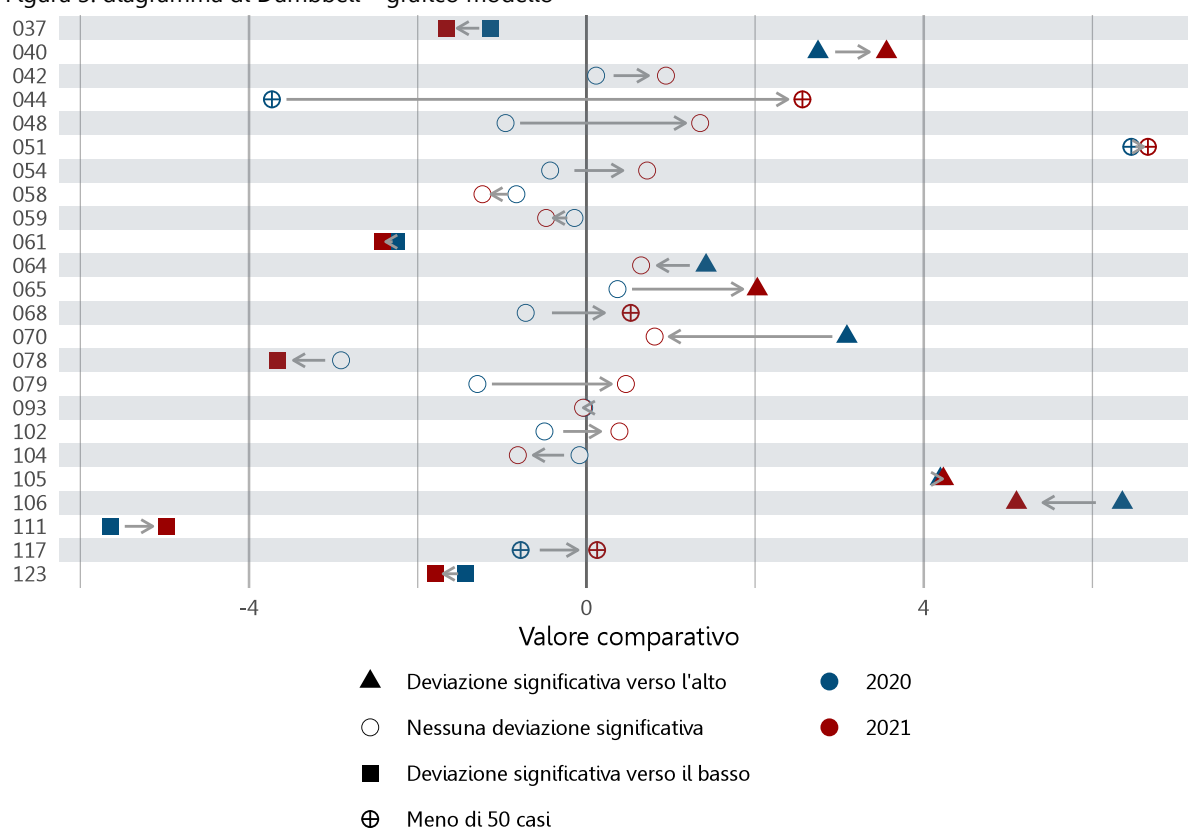
Figura 3: diagramma di Dumbbell – grafico modello
