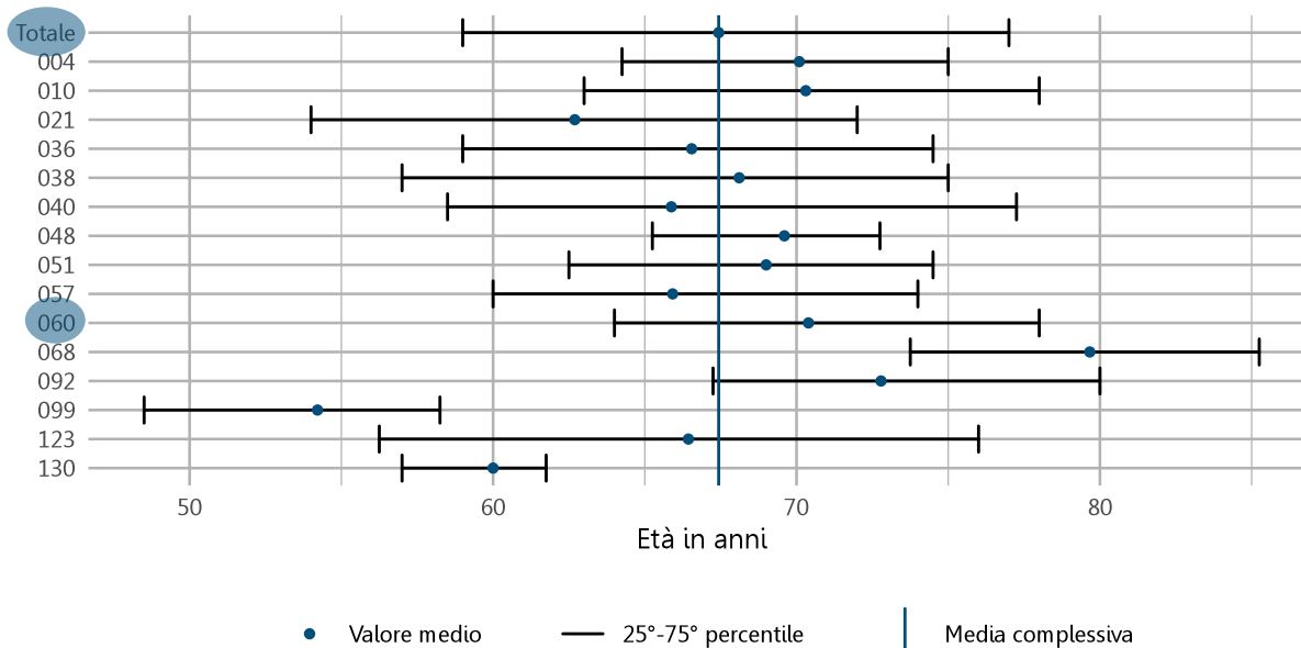
Figura 7: esempi di lettura per i tipi di grafico utilizzati: box-plot semplificato – variabili metriche (confronto tra le cliniche)
